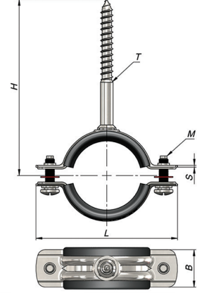
Lastiksiz sıkma ölçüsü / Clamping range without rubber
