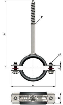
Lastiksiz sıkma ölçüsü / Clamping range without rubber
