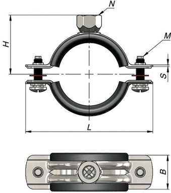
Lastiksiz sıkma ölçüsü / Clamping range without rubber
